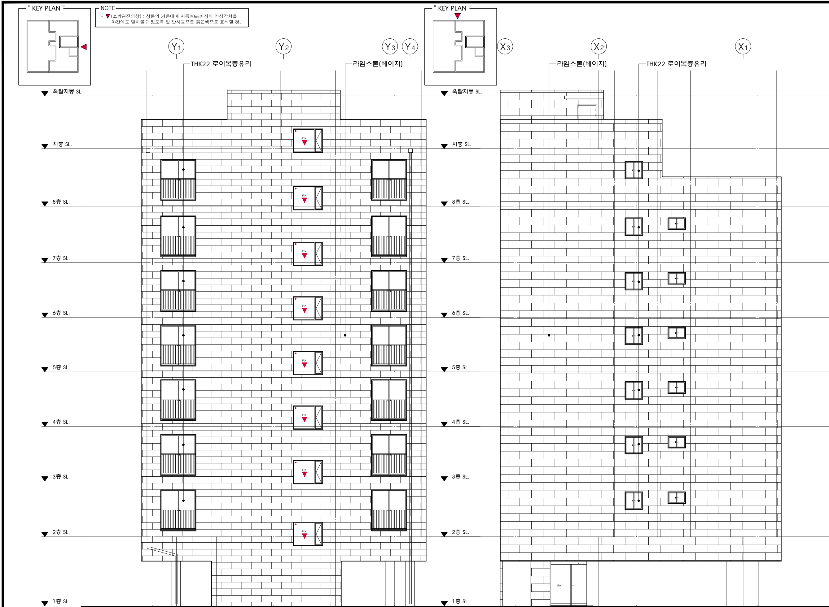
1 정 면 도 축척 - A3 : 1/120
